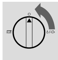
Schritt 15: (Reinigen/Abkühlen) Heißwasser-Bezug stoppen. Drehknebel nach oben drehen. Das Gerät ist betriebsbereit. HINWEIS: Das Gerät leitet überschüssiges Wasser über ein Rückführungssystem in den Wassertank zurück!
