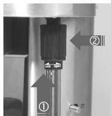
① Edelstahl-Hülse zum Aufstecken am Schaft fassen und auf die Düse aufstecken. ② Anschließend nach links drehen und verriegeln.
