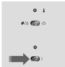
Schritt 5: Gerät einschalten. Die Betriebs-Kontrolllampe leuchtet dauerhaft. Das Gerät heizt auf, während dieser Zeit leuchtet die rote Temperatur-Kontrolllampe dauerhaft. Erlischt die Lampe, ist das Gerät betriebsbereit.
